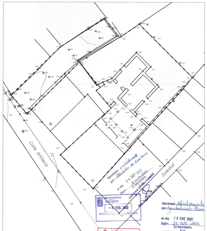
TOPOGRAFICO DE PARCELAS E:1/200
